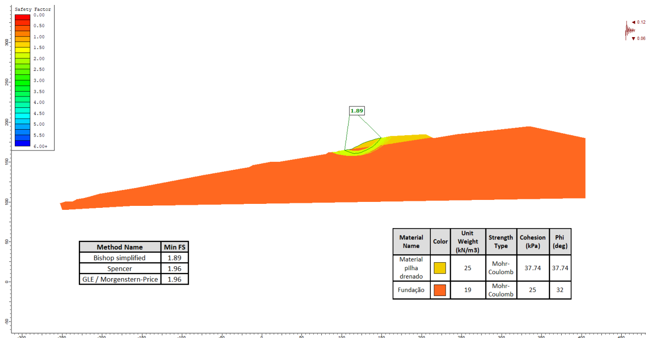
• Figura 6-19: Pseudoestática
