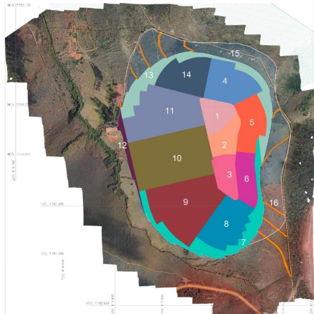
Figura 6-12: Bacias de contribuição da pilha noroeste
