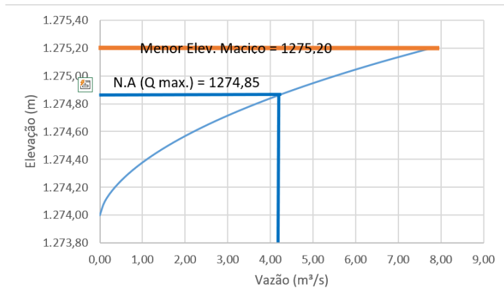
Figura 6-33: Curva Cota x Descarga do extravasor da Barragem Aredes
