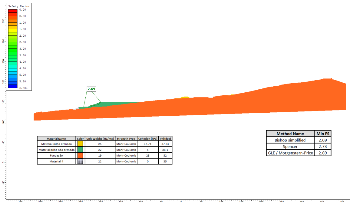
figura 6-15: Seção não drenada
