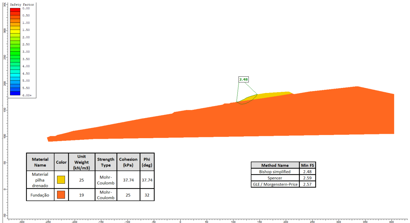
Figura 6-17: seção drenada
