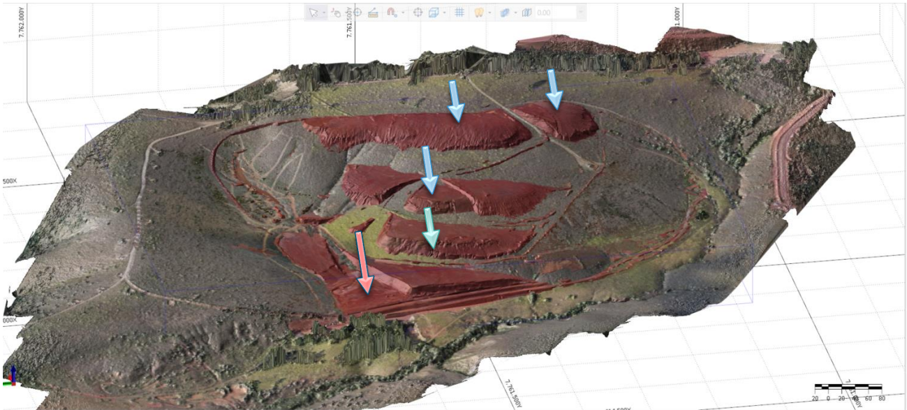
Figura 6-4: área de compactação (seta rosa) e bota espera (seta azul) na pilha noroeste. Imagem de início de novembro de 2023.
