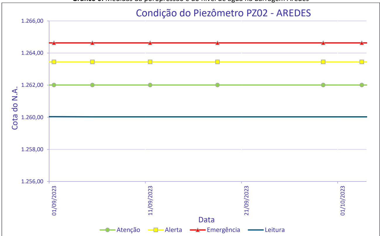
Gráfico 6: Medidas da poropressão e do nível de água na Barragem Aredes
