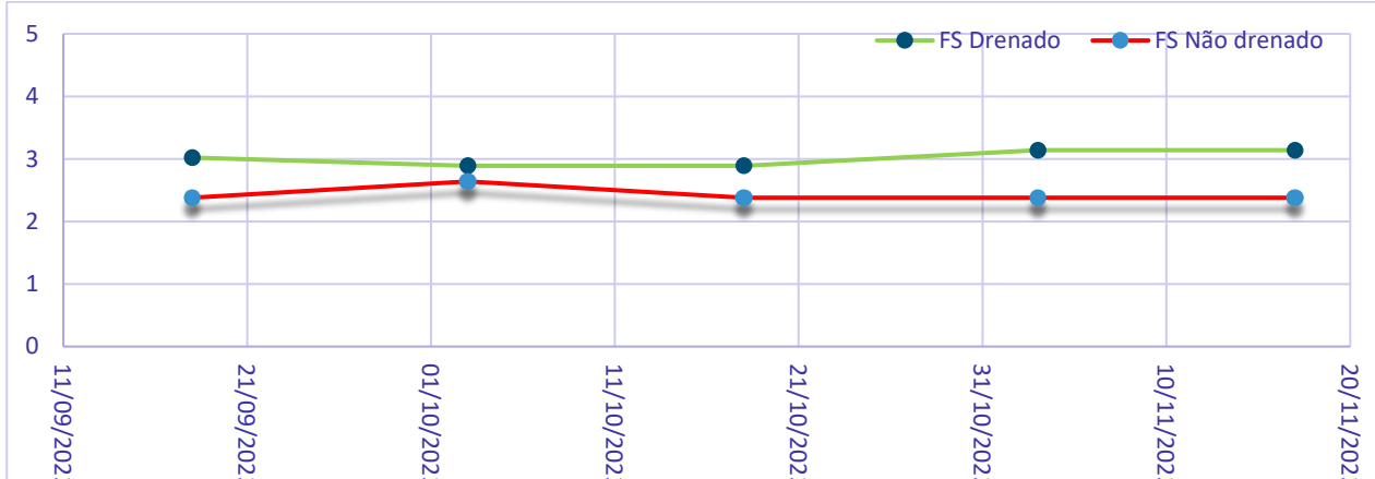
Gráfico 5: Fator de segurança do trimestre na Barragem Aredes
