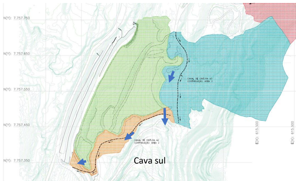
Figura 6-30: Direção do fluxo hídrico a montante na barragem Aredes
