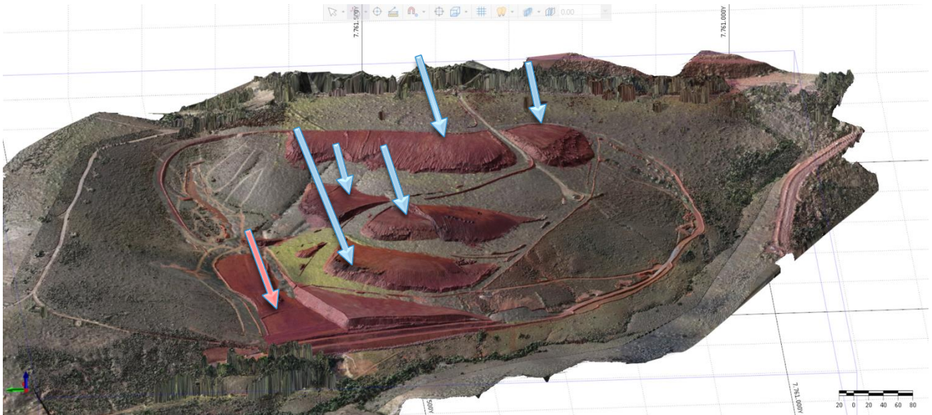
Figura 6-6: Área de compactação (seta rosa) e bota espera (seta azul) na pilha noroeste. 10/10/2023
