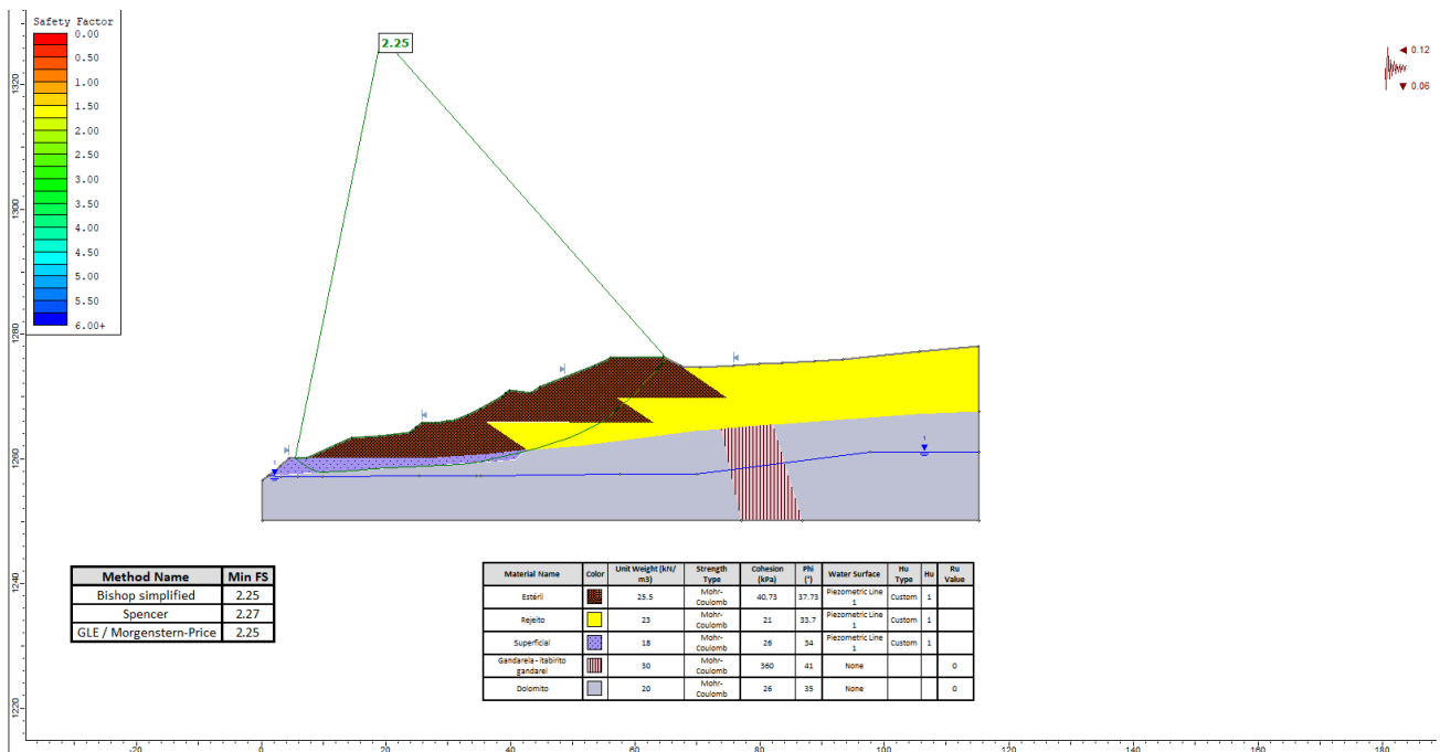
Figura 6-23: Pseudoestático (FS min: 1.10)
