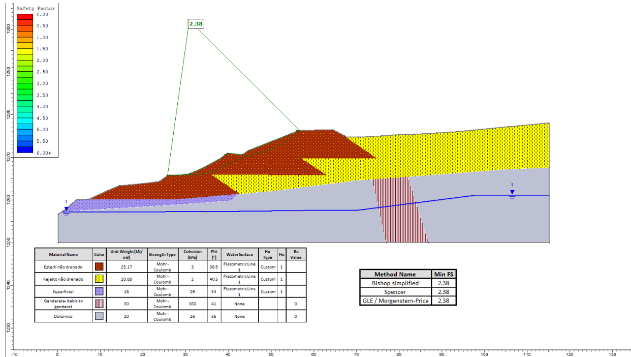
Figura 6-21: Condição não drenada. FS Min: 1,3
