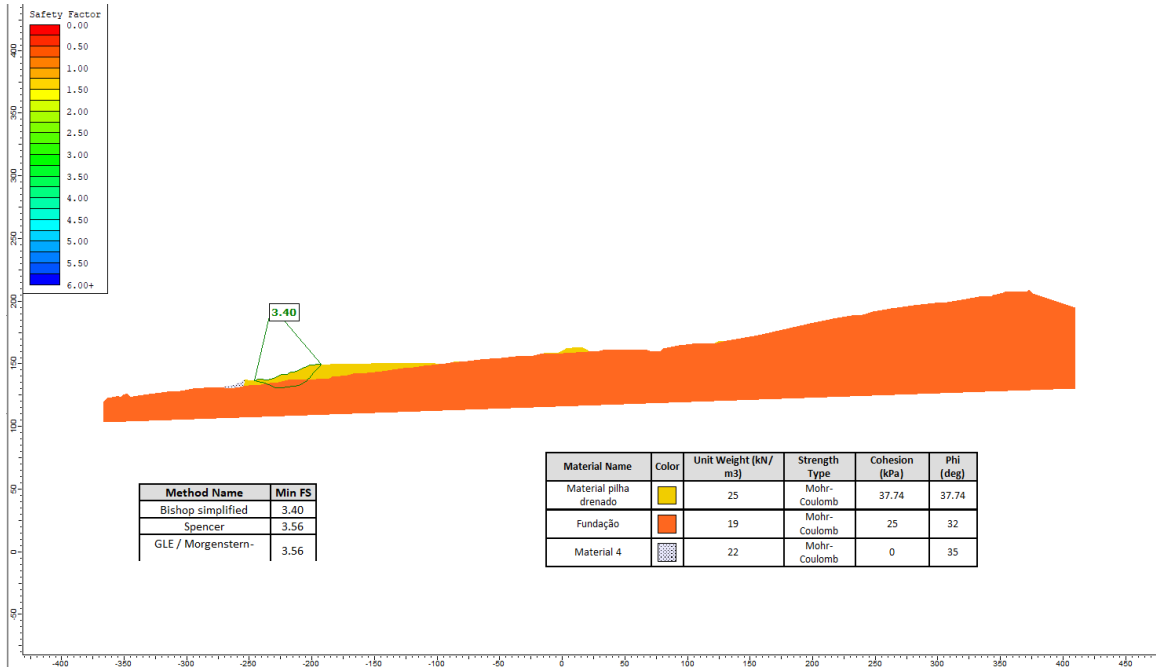
Figura 6-14: Seção drenada
