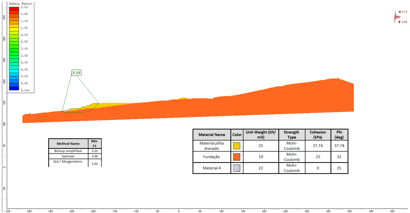
Figura 6-16: Seção pseudo-estáticas.
