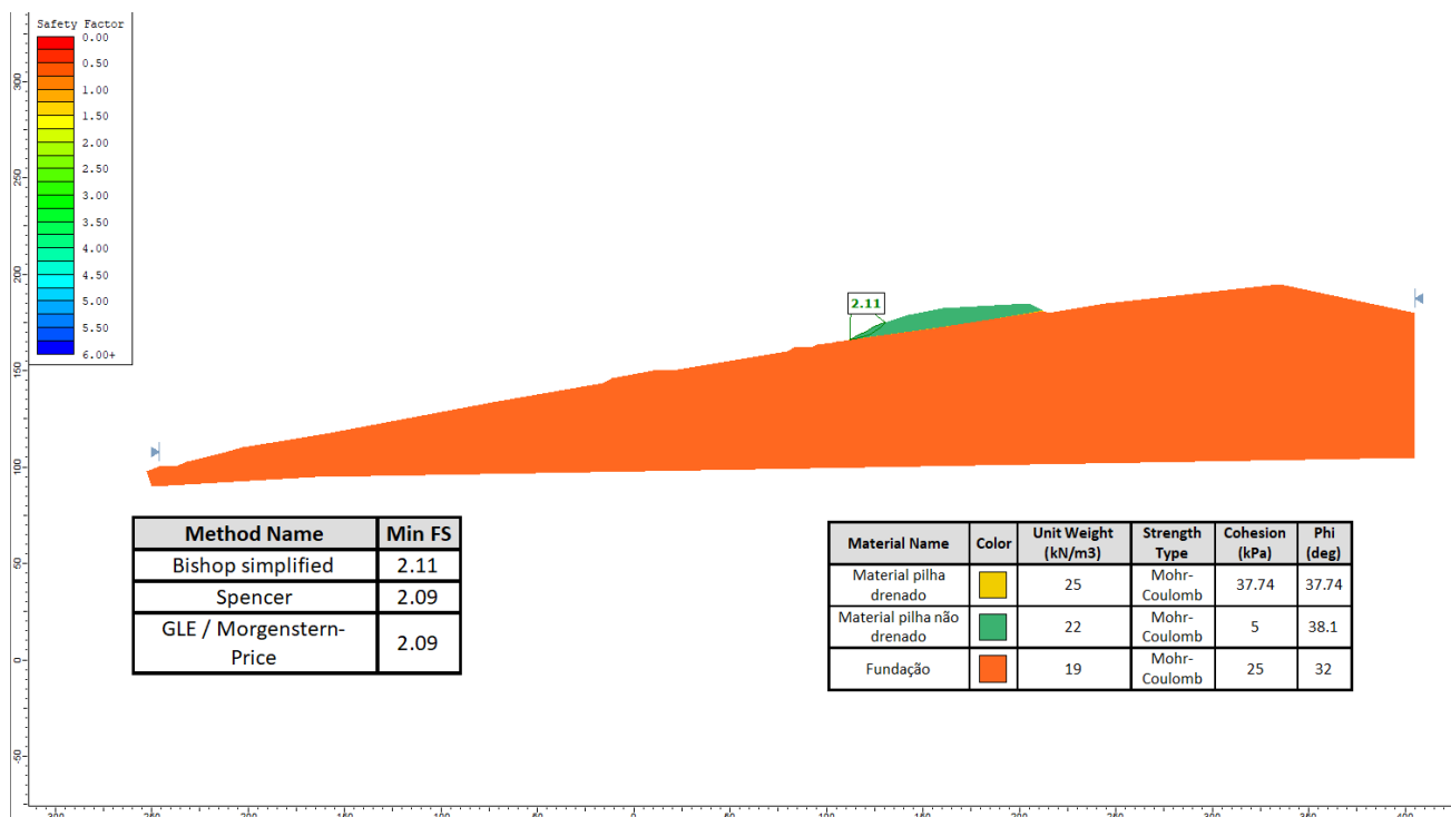
Figura 6-18: Seção não drenada
