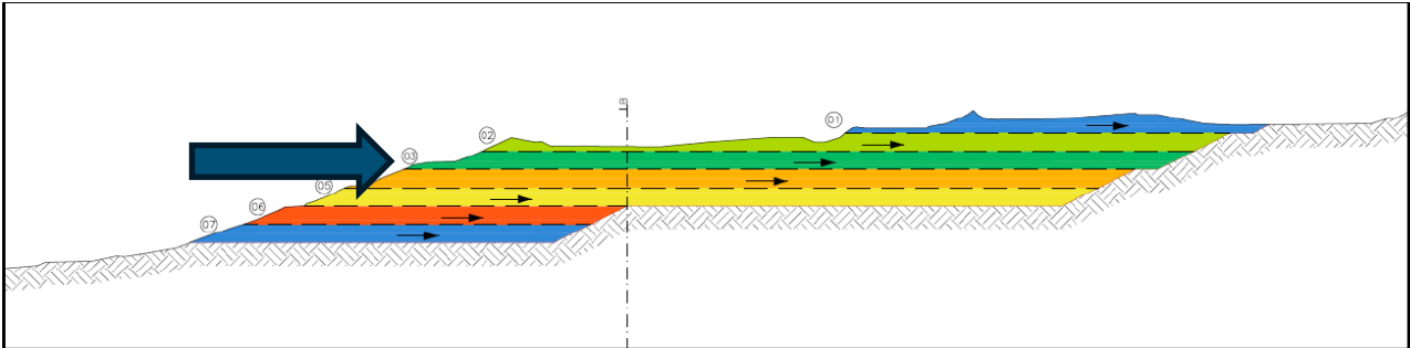
Figura 6-29: Etapa atual do processo de remoção da Barragem Central
