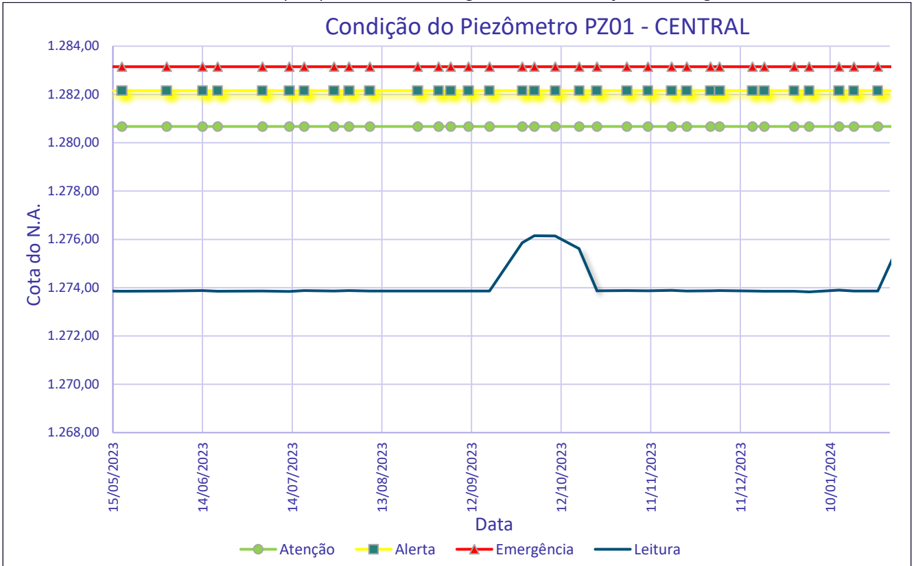
Gráfico 3: Medidas da poropressão e nível de água na instrumentação da Barragem Central.
