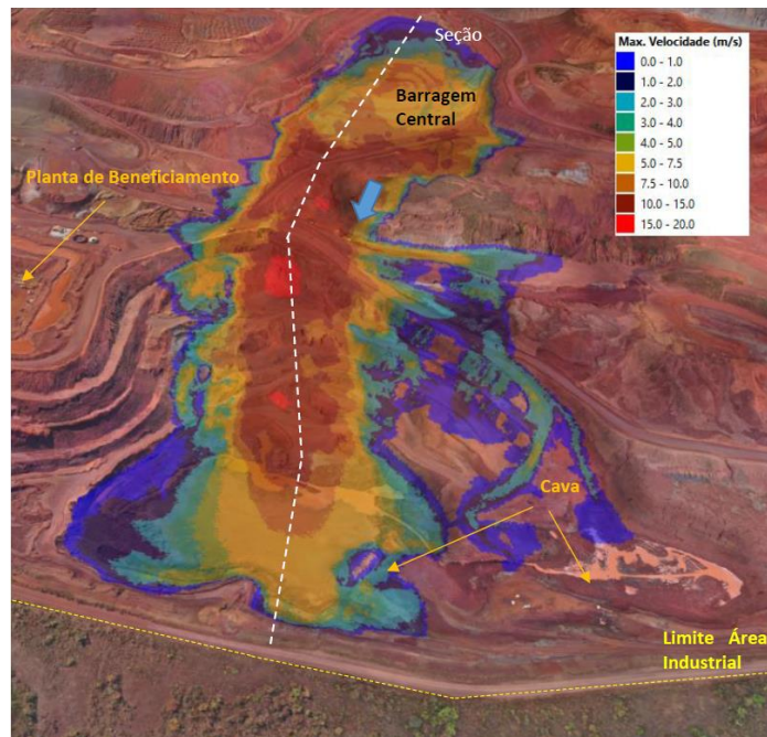
Figura 6-24: Mancha de ruptura hipotética atualizada da barragem Central.
