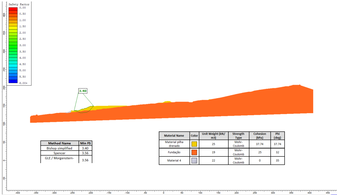
Figura 6-16: Seção drenada
