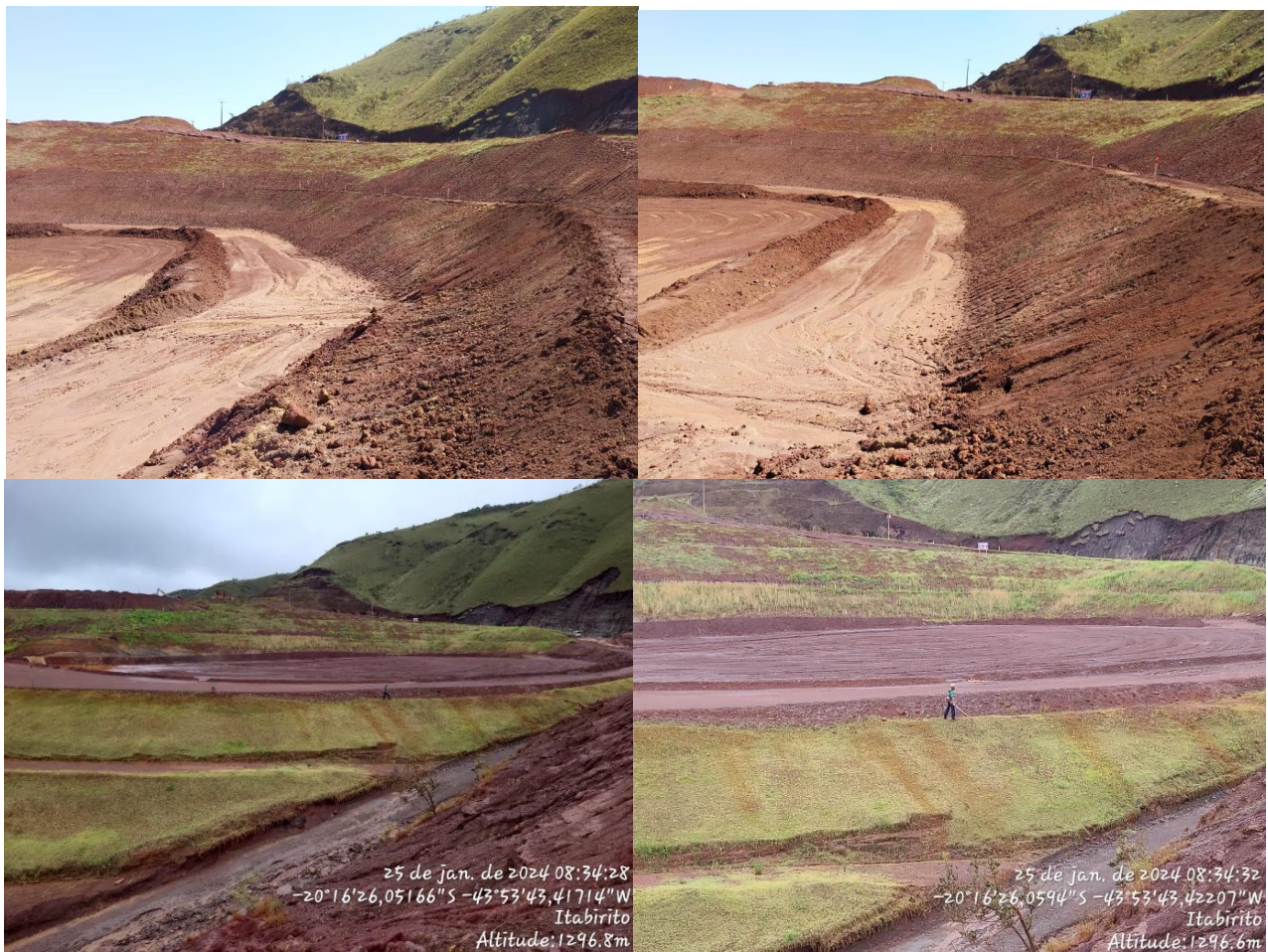
Figura 6-1: Plantio de vegetação no talude remanescente na Barragem Central. As duas primeiras fotos indicam o reservatório no início do plantio e as duas últimas fotos a atual situação da vegetação no talude remanescente.
