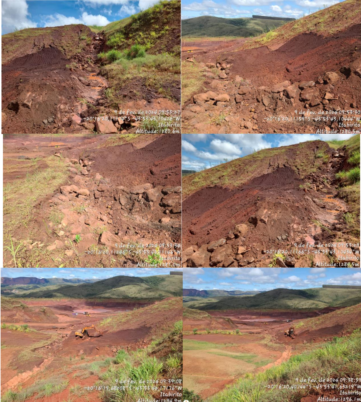
Figura 5-4: Melhoria no sistema de drenagem da Estrutura e correções de erosões na ombreira direita da estrutura.
