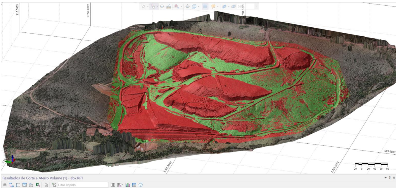
Figura 6-4: Volume trimestral depositado na pilha noroeste
