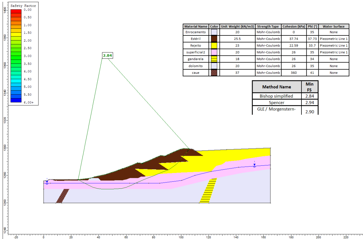
Figura 6-21: Condição drenada FS Min: 1,5
