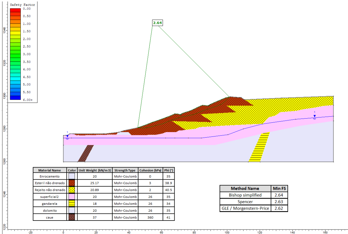
Figura 6-20: Condição não drenada. FS Min: 1,3
