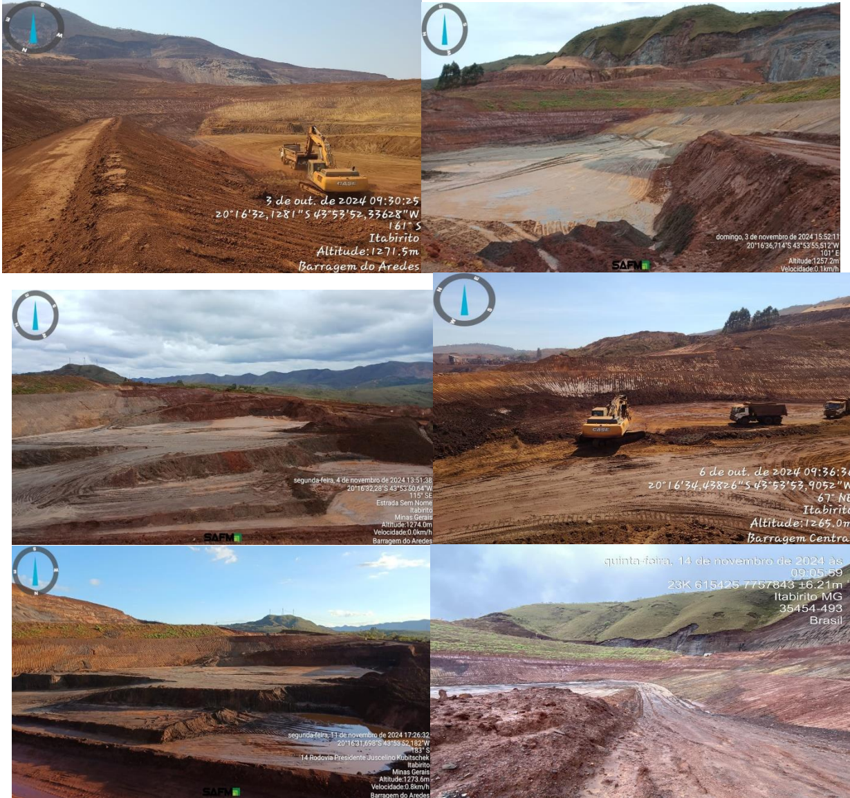
Figura 7: Remoção do barramento e rejeito ao longo do processo de descaracterização
