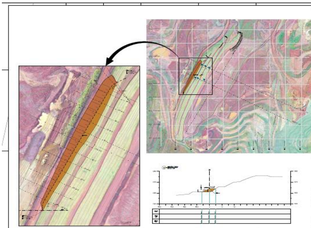
Figura 6-28: Reforço realizado na Barragem Aredes
