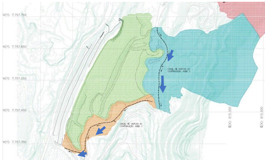
Figura 6-53: Direção do fluxo hídrico a montante da antiga Barragem Aredes
