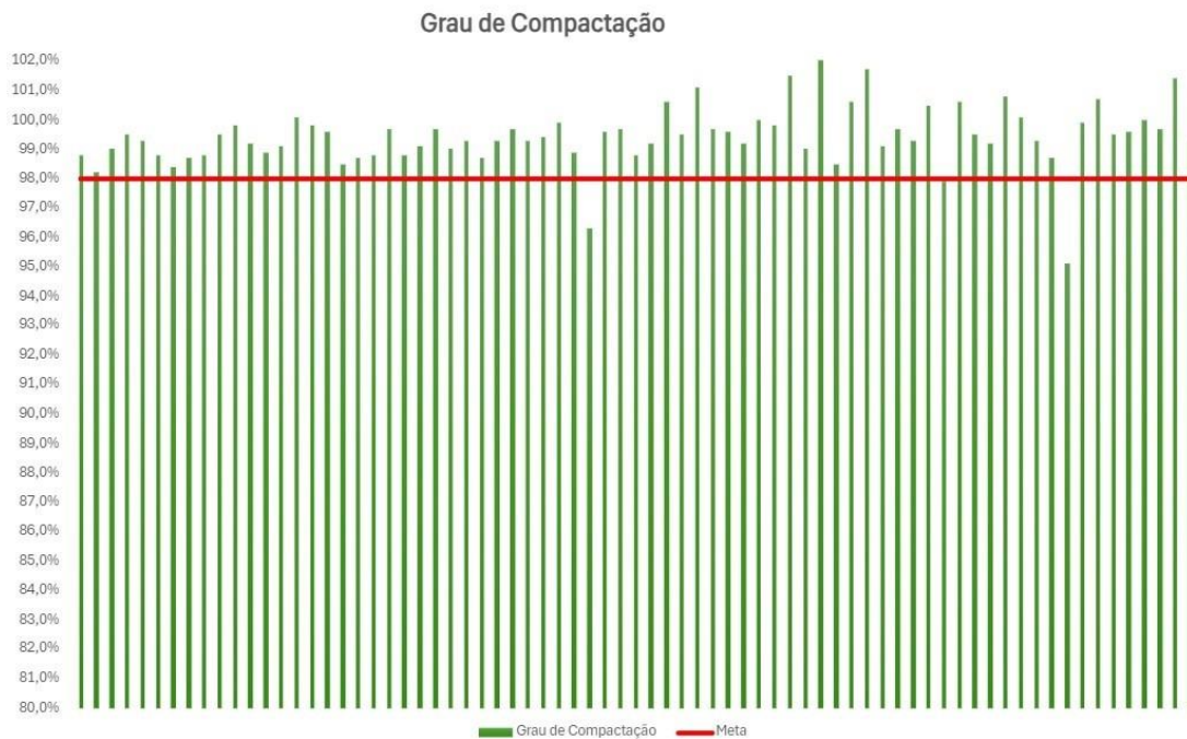
Figura 8: Grau de compactação obtido na pilha noroeste ao longo do trimestre. Apenas aquelas acima de 98% são aprovados.
