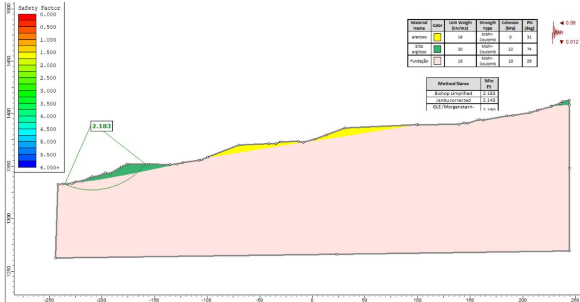
Figura 6-18: Seção pseudoestática da pilha ascendente noroeste.
