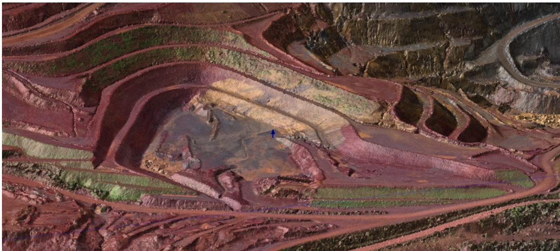
Figura 6: Continuidade da remoção do maciço e rejeito remanescente. Outubro e novembro, respectivamente
