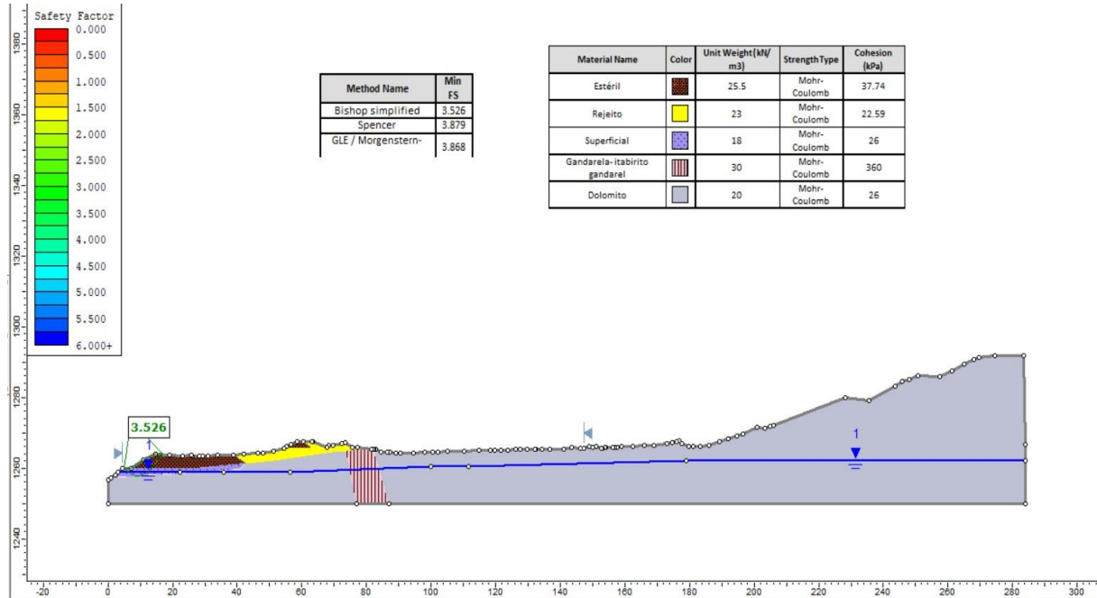
Figura 6-24: Condição drenada FS Min: 1,5
