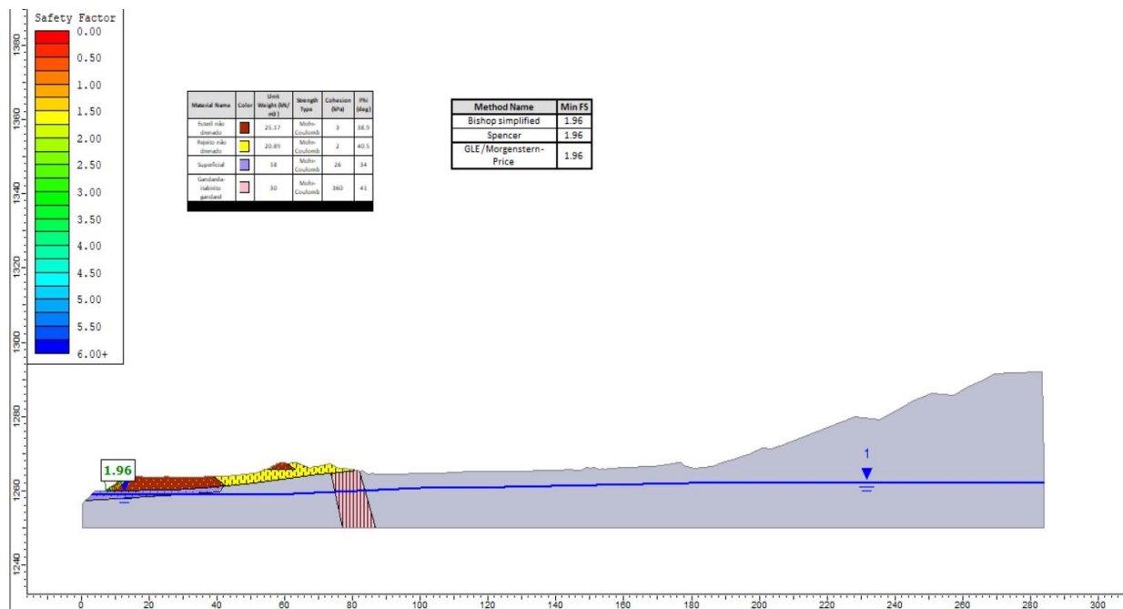
Figura 6-23: Condição não drenada. FS Min: 1,3
