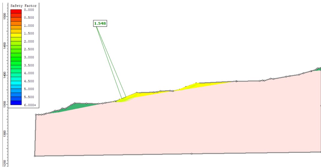
figura 6-17: Seção drenada do bota espera (praças 04 e 7)
