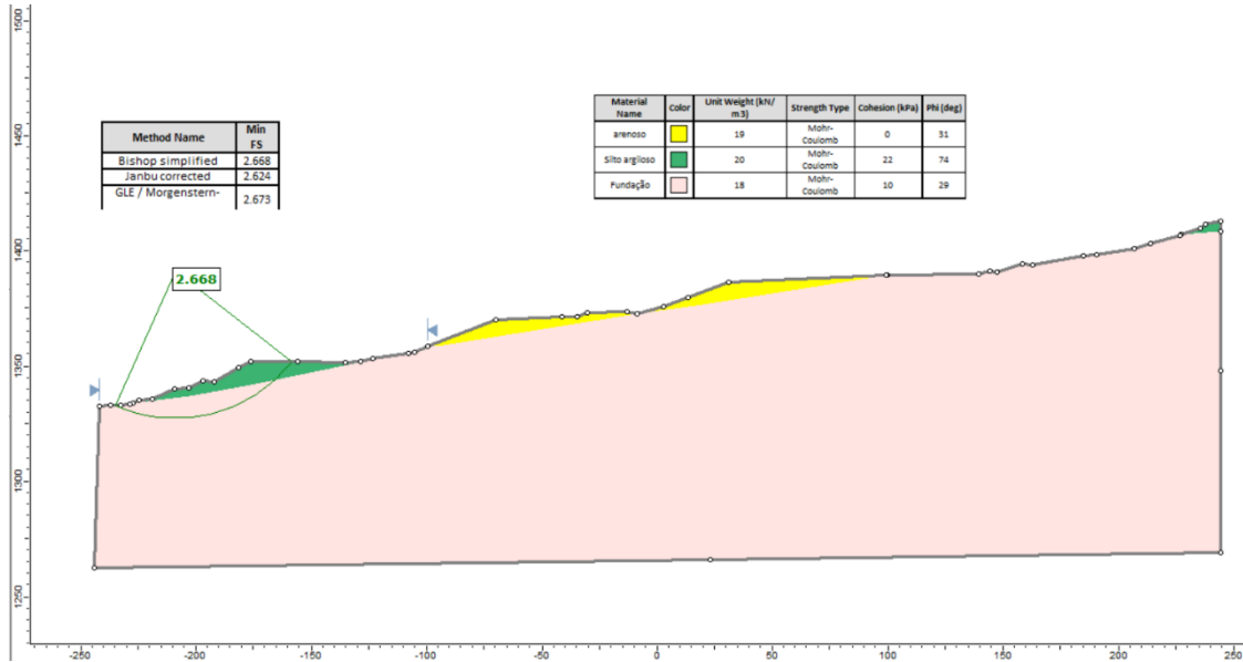
Figura 6-16: Seção drenada praça 01
