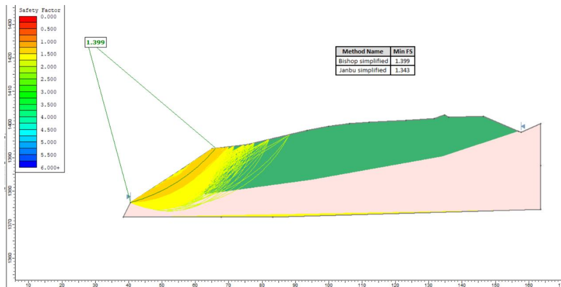
Figura 19: Seção não drenada na praça 10
