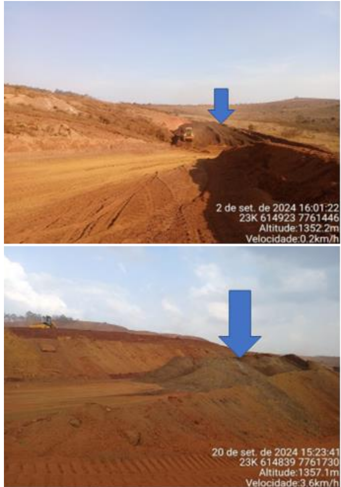
Foto 10: basculamento de estéril nas bermas das praças 03 e 01, respectivamente.
