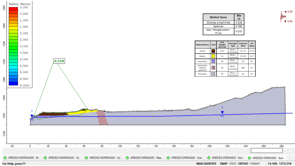
Figura 6-27: Pseudoestático – Detonação (FS min: 1.10)
